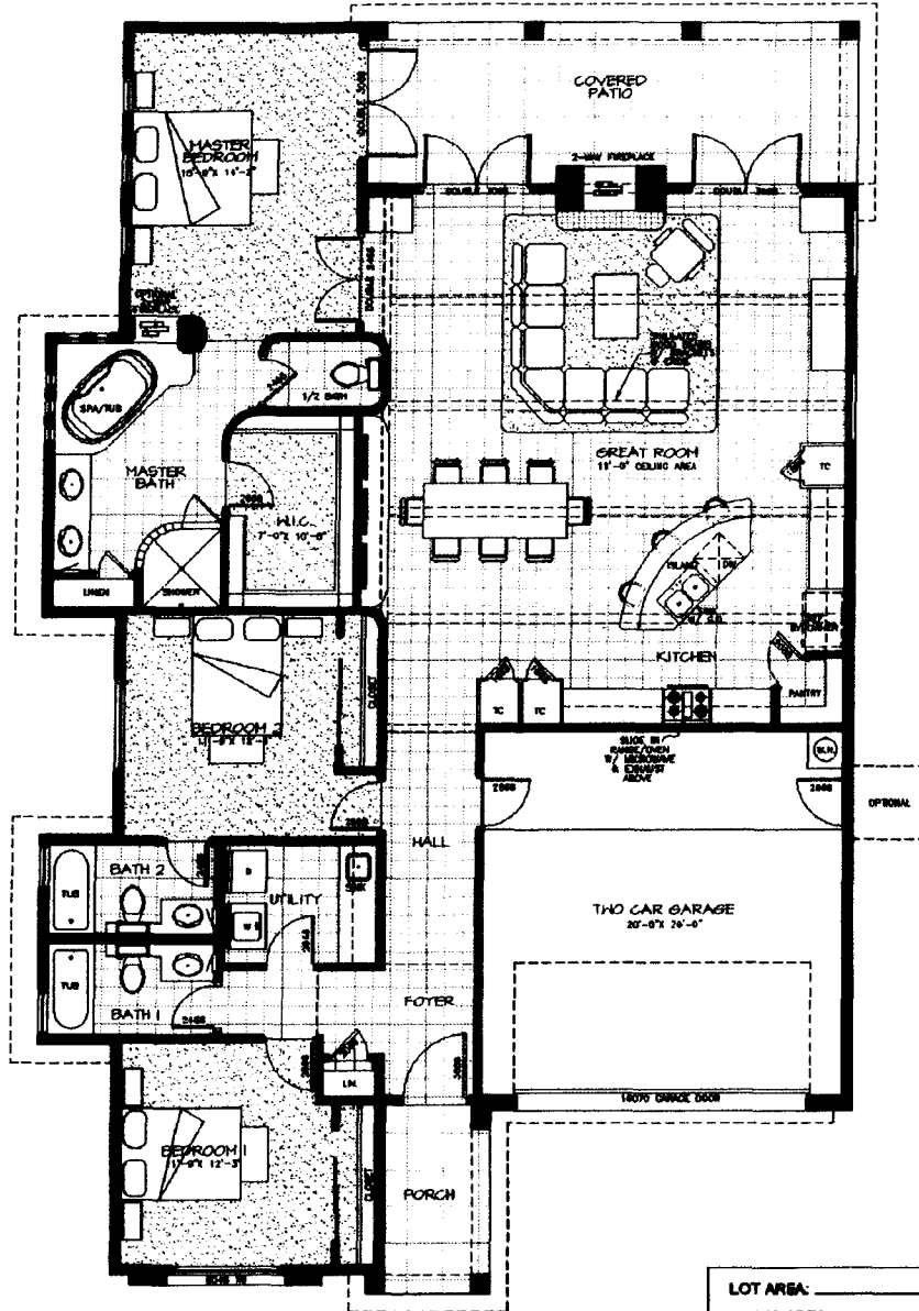
OPTIONAL GOURMET KITCHEN SCALE: 1/4" = 1'-0"
